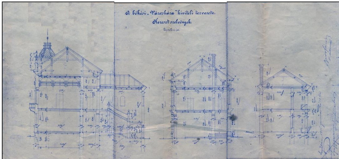
A békési Városháza kiviteli tervezetének kereszt-szelvényei (JMM. Td.89.225.1.)
